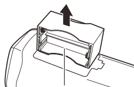
電池ケース
